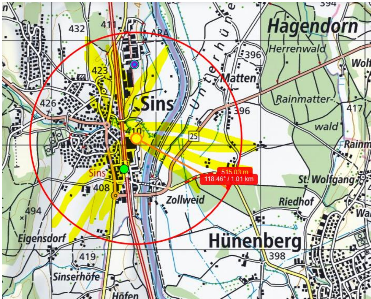
Plausibelste Sende-Richtungs-Verteilung eines so solitären Standorts
