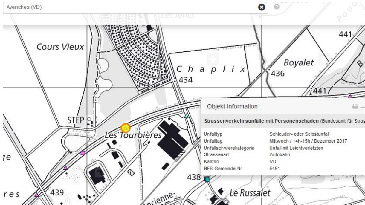
Unfallschwerpunkt, Schleuderunfall
