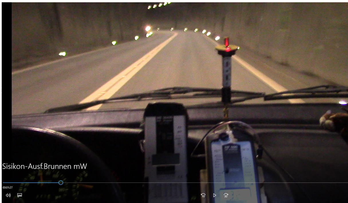
3.6 mW im Bereich des Senders (2 sec. zeitverzögerte Darstellung, in Gegenrichtung)
