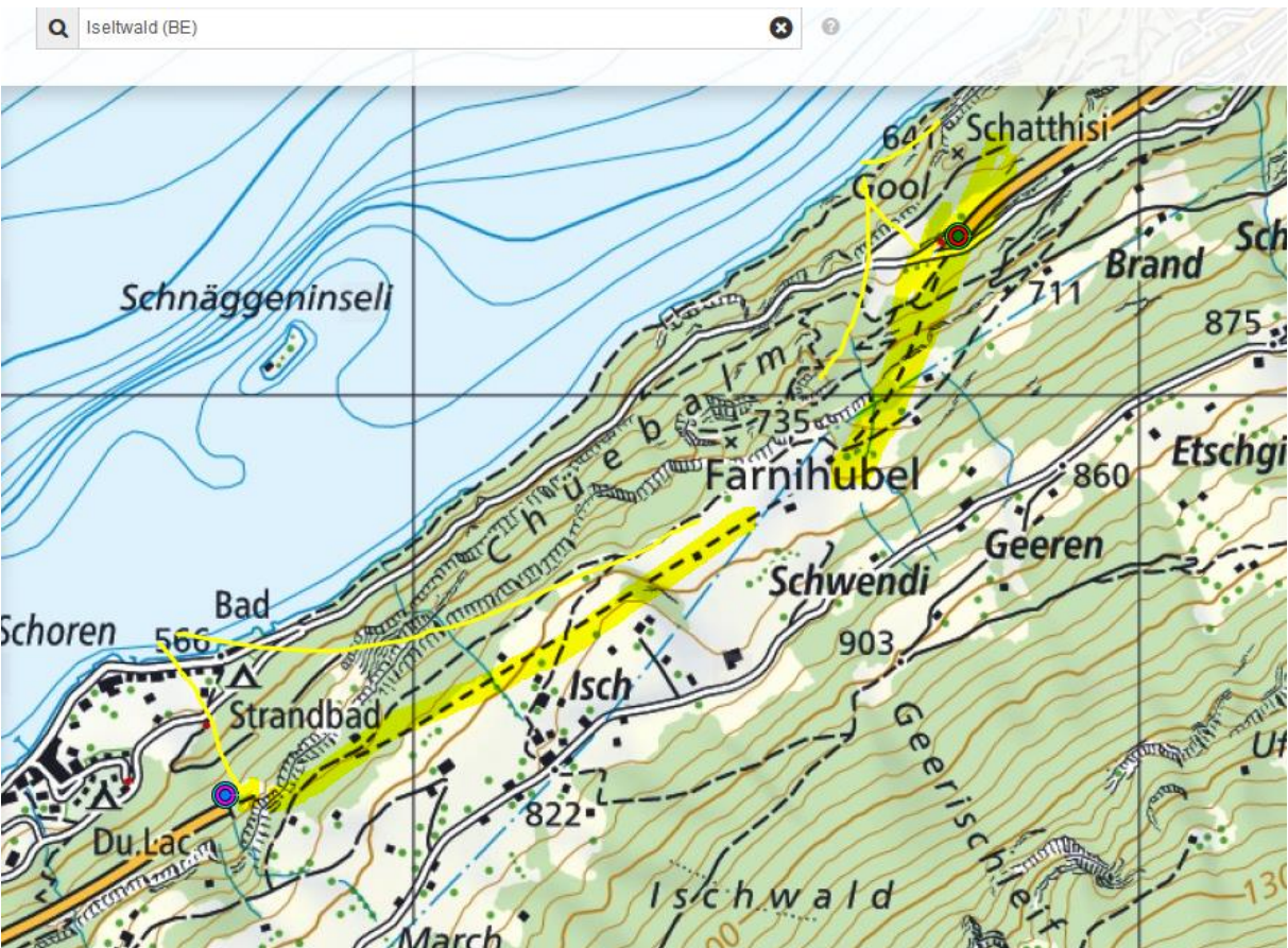
Gelbe Linie: visualisierte Sendeleistung / Belastung im Tunnelverlauf
